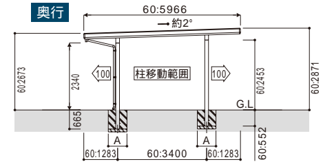
【側面図】
