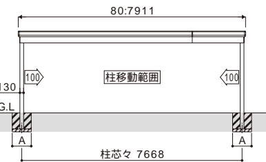
寸法図(単位mm)
